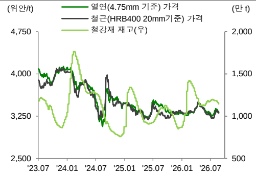
도표 22. 철강 가격 ↑, 철강재 재고 ↓
