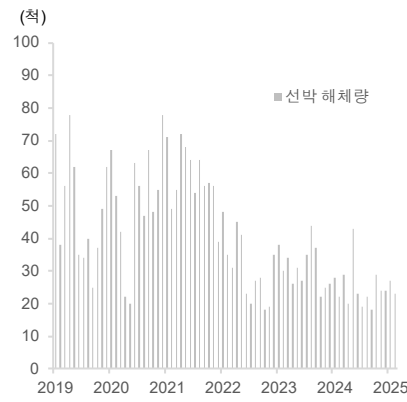
선박 해체량(최근4년내)
