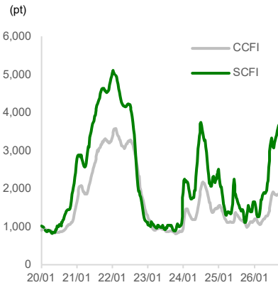
SCFI, CCFI(컨테이너운임지수)
