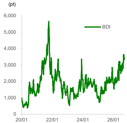
BDI(벌크선 운임지수)
