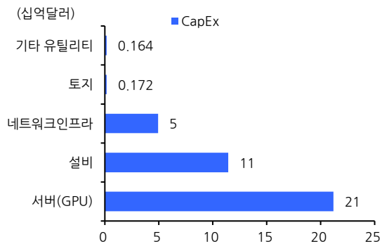
〈그림19〉 AIDC 1GW 기준 초기 투자비
