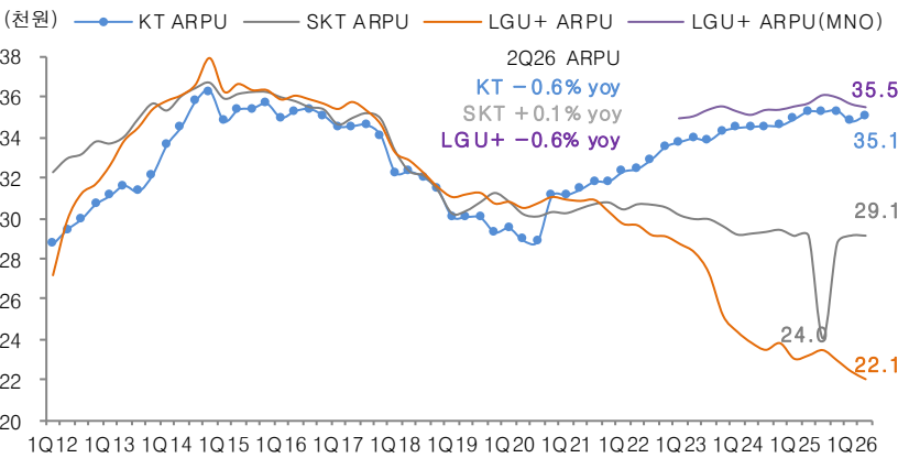
그림 7. 무선 ARPU
