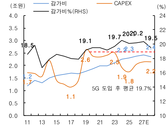
그림 13.CAPEX/감가비 전망
