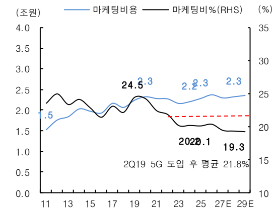
그림 11.마케팅비 전망
