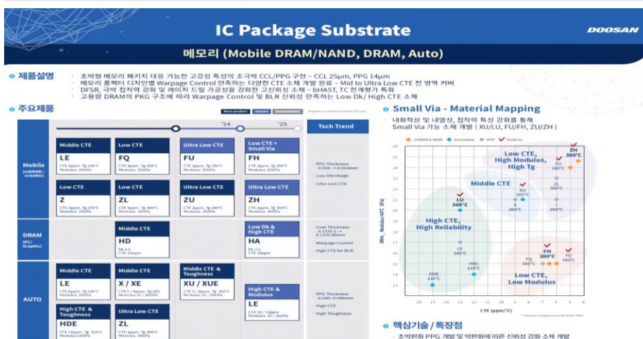
그림7 두산 전자BG 메모리 기판용 CCL 라인업
