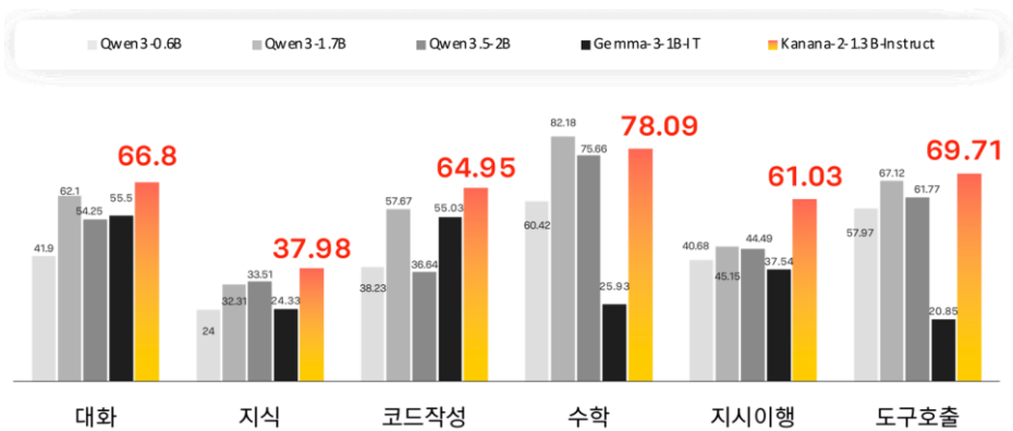
그림 3. Kanana 2-1.3B 모델 벤치마크 비교
