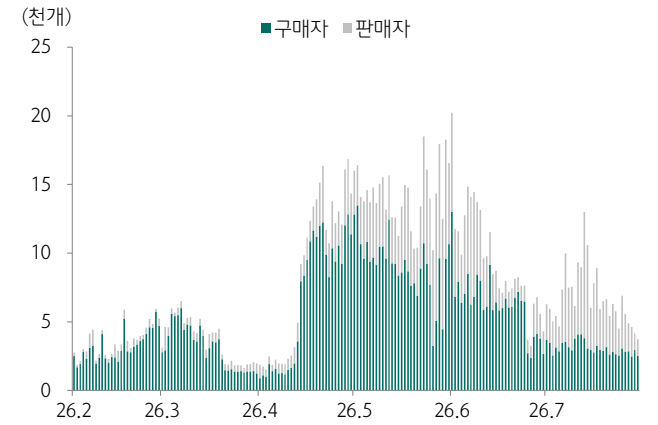
도표 18. x402 구매자/판매자 추이
