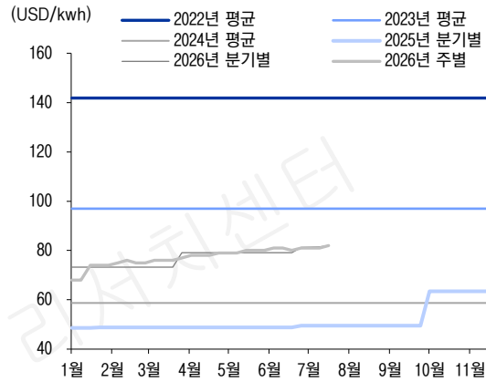
그림6 파우치형 배터리 가격 추이
