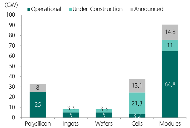
도표 37. 현재 미국 태양광 모듈 설비 규모는 약 65GW
