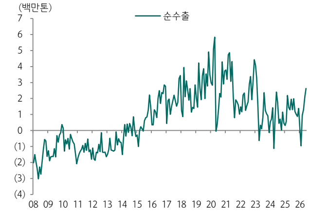
도표 124. 중국 6월 석유제품 순수출 MoM +27%
