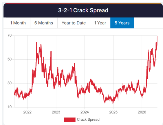
도표 1. 미국 3-2-1 정제마진 역사적 최대치를 기록 중
