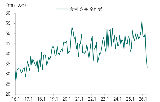
도표 12. 중국 원유 수입량 추이
