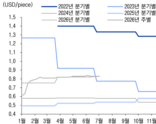
그림7 원통형 삼원계 배터리 가격 추이
