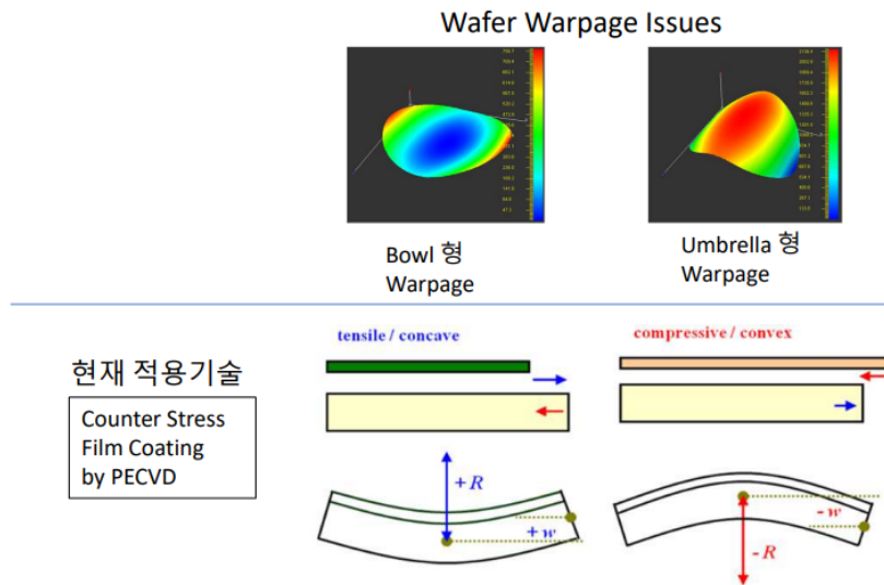
그림 2. Wafer warpage 이슈와 종류
