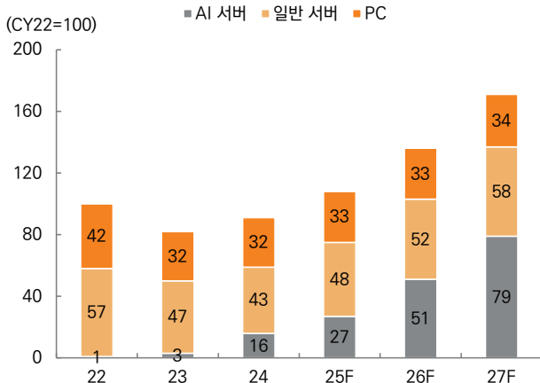
그림 4. 이비덴 FC-BGA 수요처별 수요 전망
